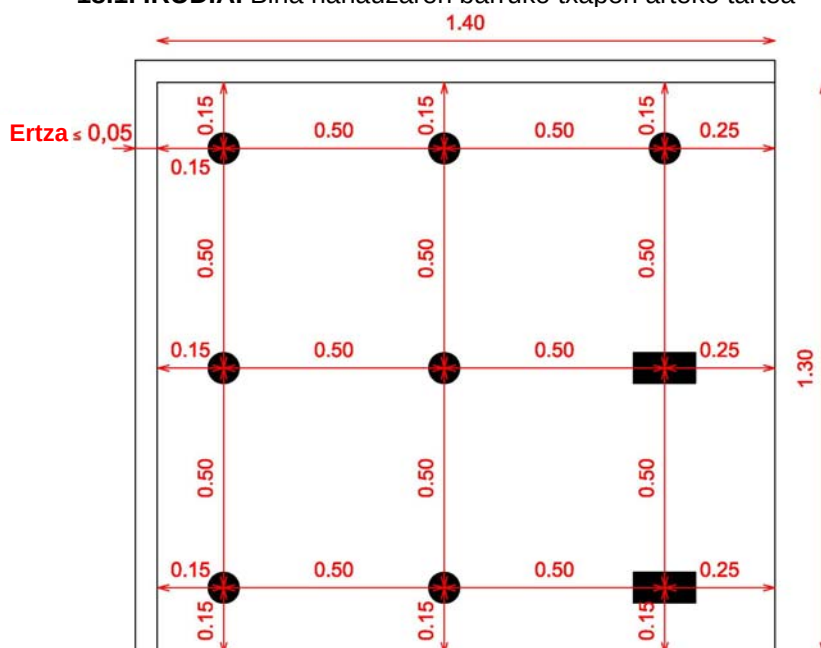
18.1. IRUDIA. Birla harlauzaren barruko txapen arteko tarteak
